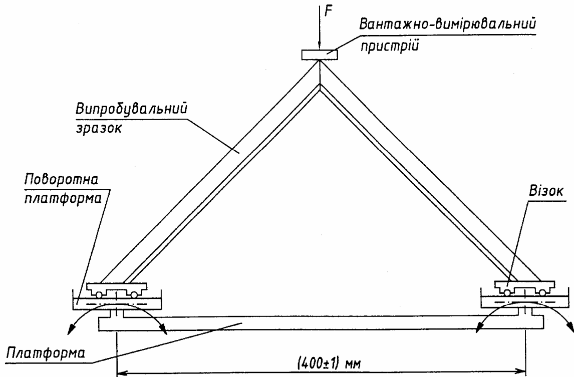
Схема випробувань кутових з'єднань
