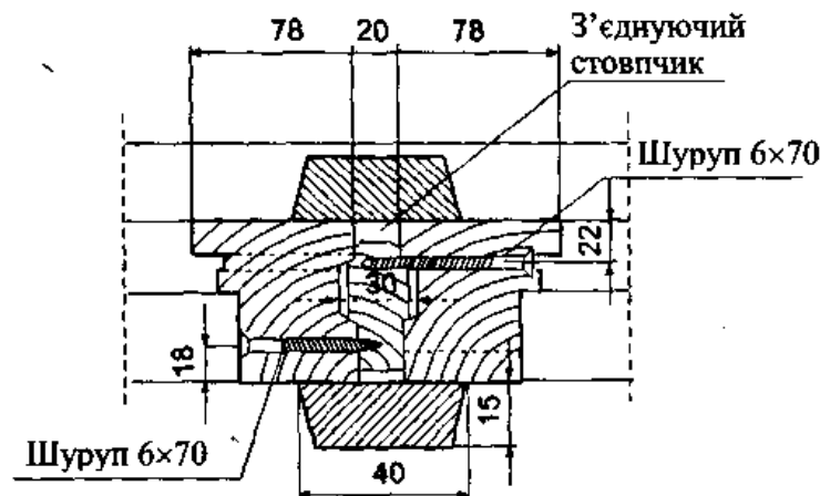
Рисунок 17 – Приклад з'єднання дерев'яних віконних блоків
