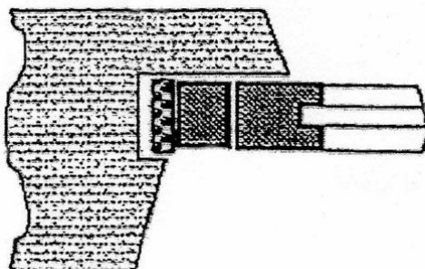
Рисунок 7 – Використання розширювальних профілів для оптимізації товщини ізоляційного шва
