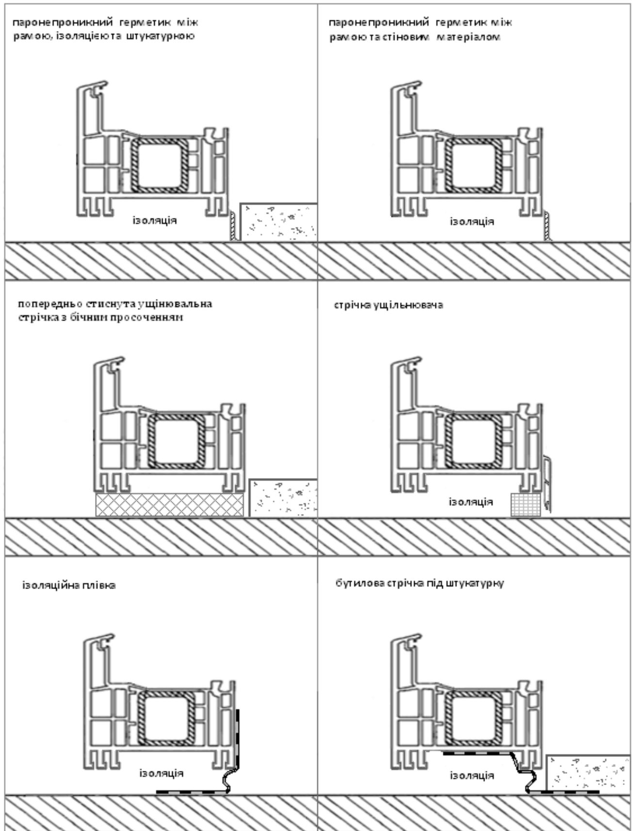
Рисунок 25 – Приклади герметизації з'єднувальних швів з боку приміщення залежно від вибраного виду ізоляційного матеріалу на прикладі віконних блоків з ПВХ
