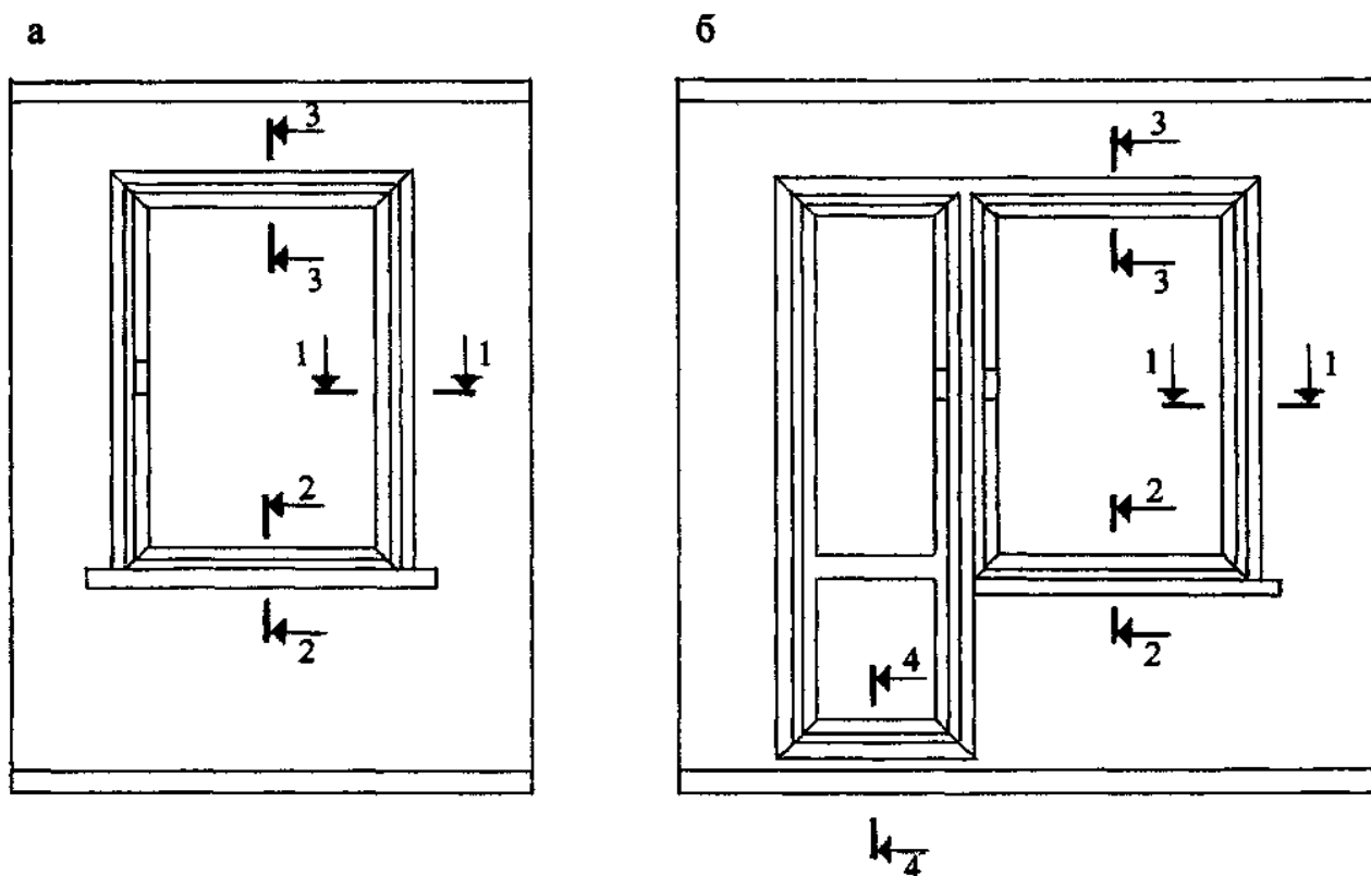
а – віконного блока; б – блока балконної двері
